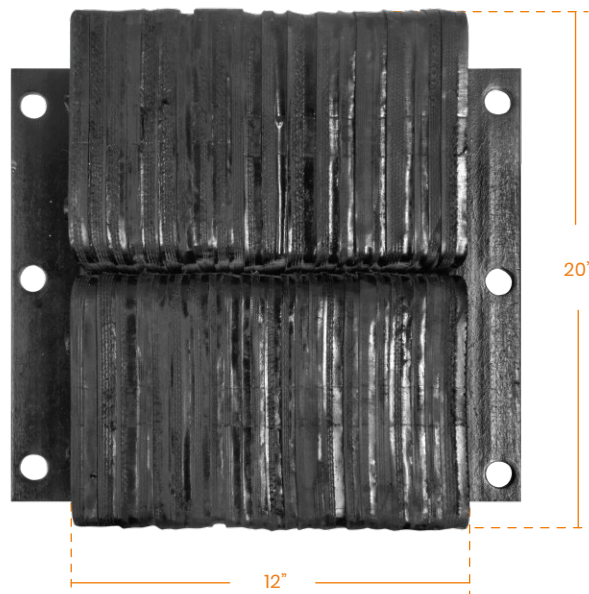
TOPE DOBLE VERTICAL 12" X 20" Modelo 00-122045DBAA-63.
