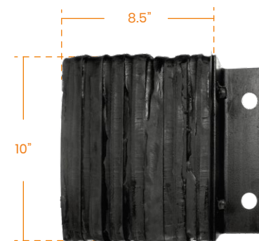
TOPE ÁNGULO-SOLERA Modelo 00-851045AS-63
